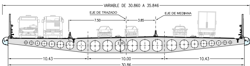
SECCION TRANSVERSAL TRAMO 10 ESCALA 1:300
