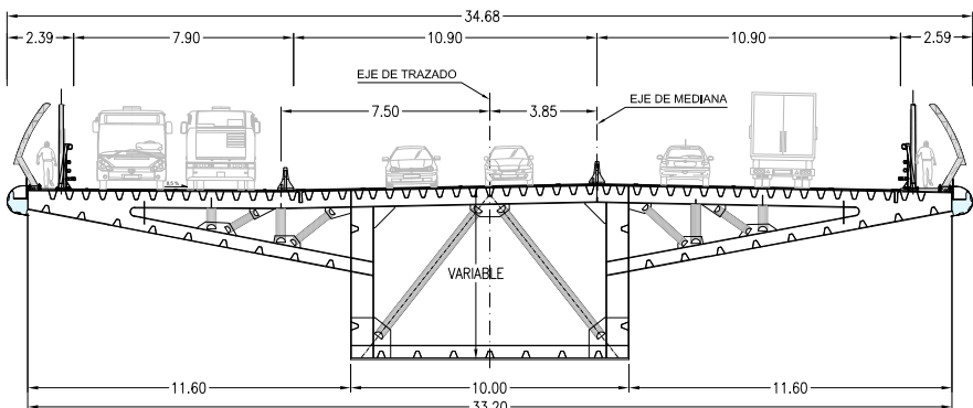
SECCION TRANSVERSAL TIPO TRAMO 3-4 ESCALA 1:300
