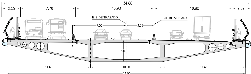
SECCION TRANSVERSAL TRAMO 8 ESCALA 1:300
