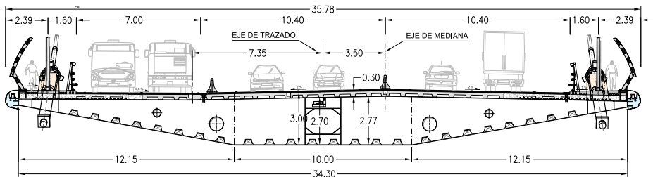
SECCION TRANSVERSAL TRAMO 6 ESCALA 1:300
