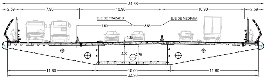
SECCION TRANSVERSAL TRAMO 2 ESCALA 1:300
