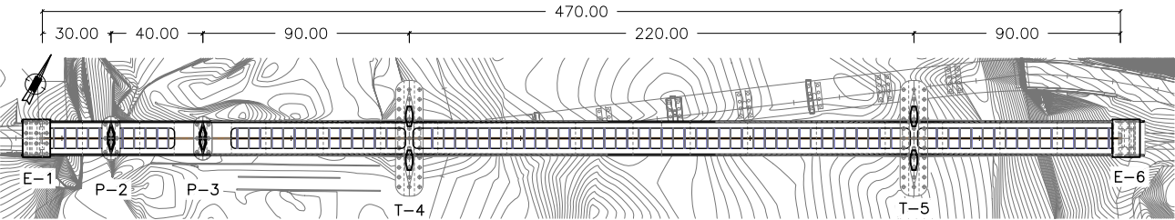
PLANTA INFERIOR ESCALA 1:3000
