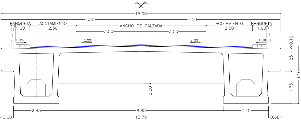
SECCIÓN TRANSVERSAL TIPO ESCALA 1:100
