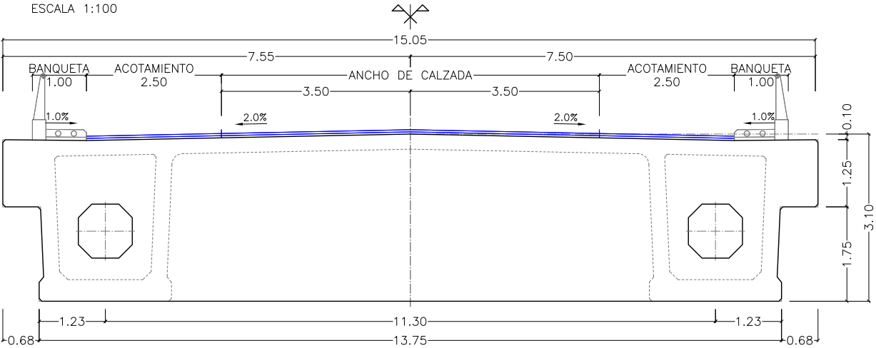
SECCIÓN TRANSVERSAL POR PILA ESCALA 1:100
