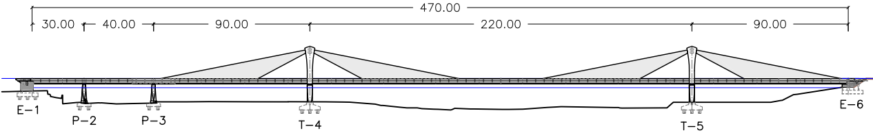
ALZADO GENERAL ESCALA 1:3000
