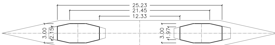
SECCION B-B ESCALA 1:350
