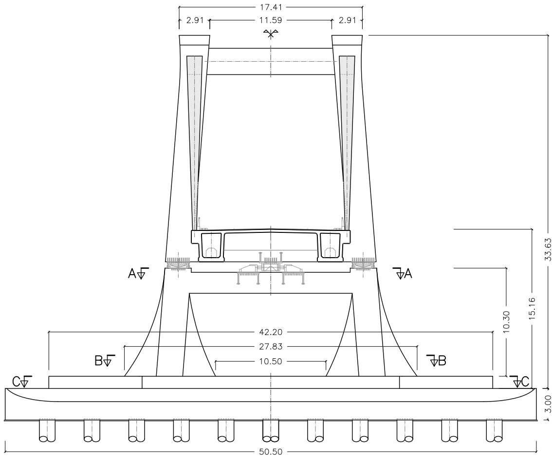
ALZADO FRONTAL DE TORRE ESCALA 1:350
