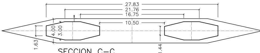
SECCION C-C ESCALA 1:350
