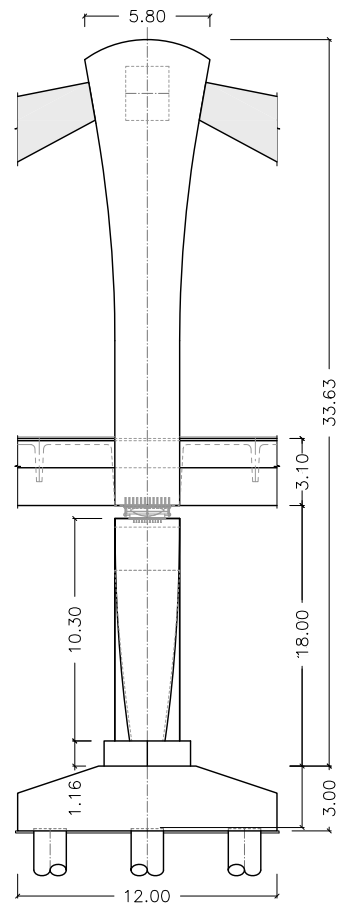
ALZADO LATERAL DE TORRE ESCALA 1:350
