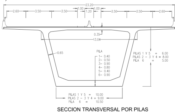
Figura 4 Sección transversal por pilas
