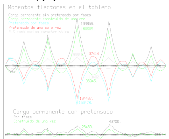
Figura 8 Resumen de esfuerzos en el tablero
