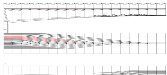
Figura 5 Esquema pretensado por P3
