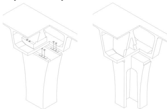
Figura 10 Esquema de empotramiento provisional con neoprenos y pretensado vertical (pilas 1, 5 y 6) y empotramiento definitivo (pilas 2, 3 y 4)
