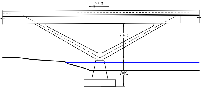
PILAS 3 Y 4. ALZADO LATERAL ESCALA 1:500
