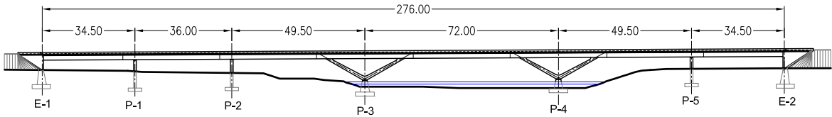
ALZADO GENERAL ESCALA 1:2000
