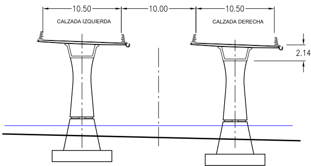
PILAS 3 Y 4. ALZADO FRONTAL ESCALA 1:500
