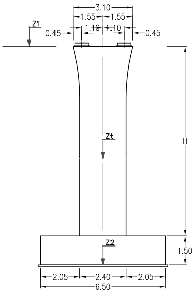
ALZADO FRONTAL. RESTO PILAS ESCALA 1:200
