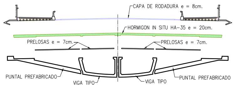
DESCOMPOSICION SECCION TRANSVERSAL ESCALA 1:250
