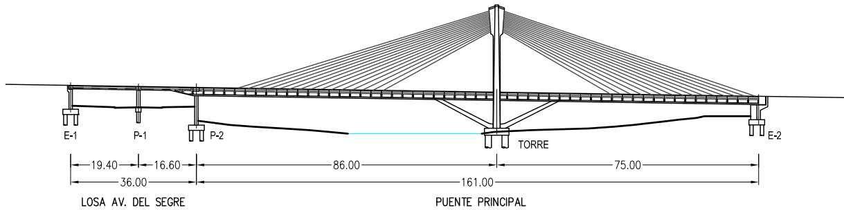
ALZADO GENERAL ESCALA 1:1500
