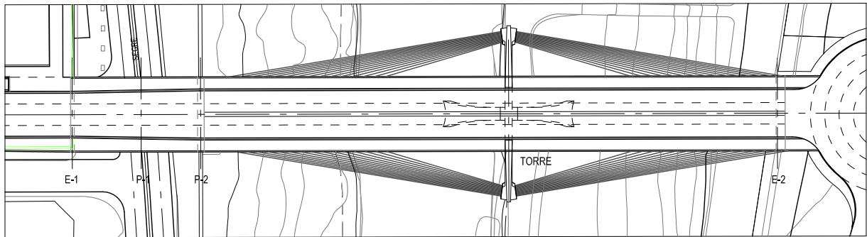
PLANTA GENERAL ESCALA 1:1500
