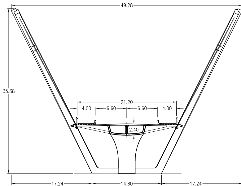
SECCION TRANSVERSAL POR PILA ESCALA 1:500
