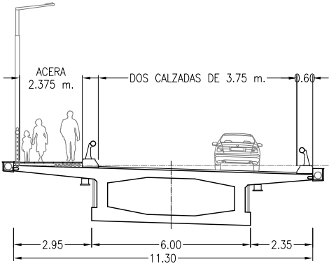
SECCION TRANSVERSAL TIPO EN RAMALES ESCALA 1:200
