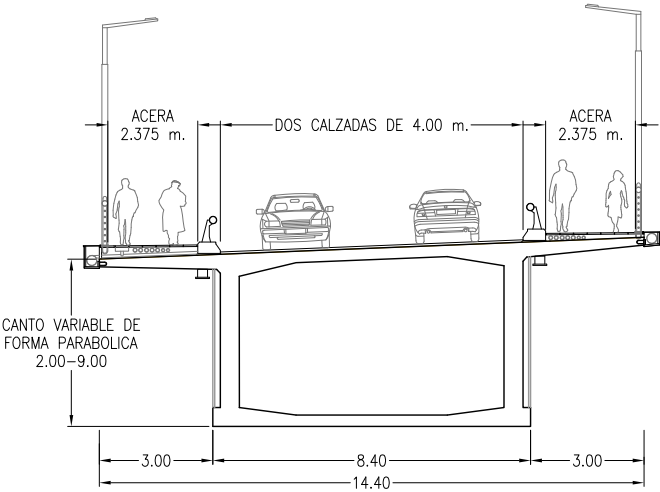
SECCION TRANSVERSAL. CANTO VARIABLE ESCALA 1:200
