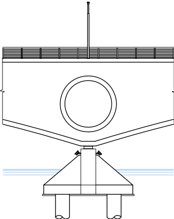
ALZADO LATERAL ESCALA 1:400
