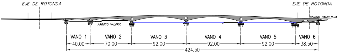
ALZADO GENERAL ESCALA 1:4000
