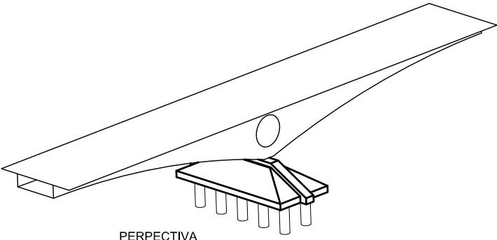
PERPECTIVA
