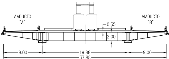
SECCION TRANSVERSAL. VIADUCTO PRINCIPAL ESCALA 1:500
