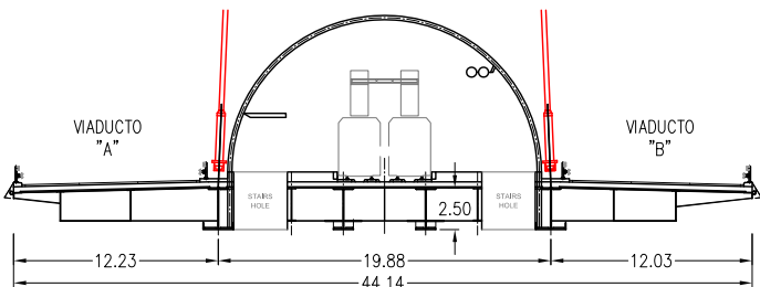
INTERSECCION ESCALA 1:500
