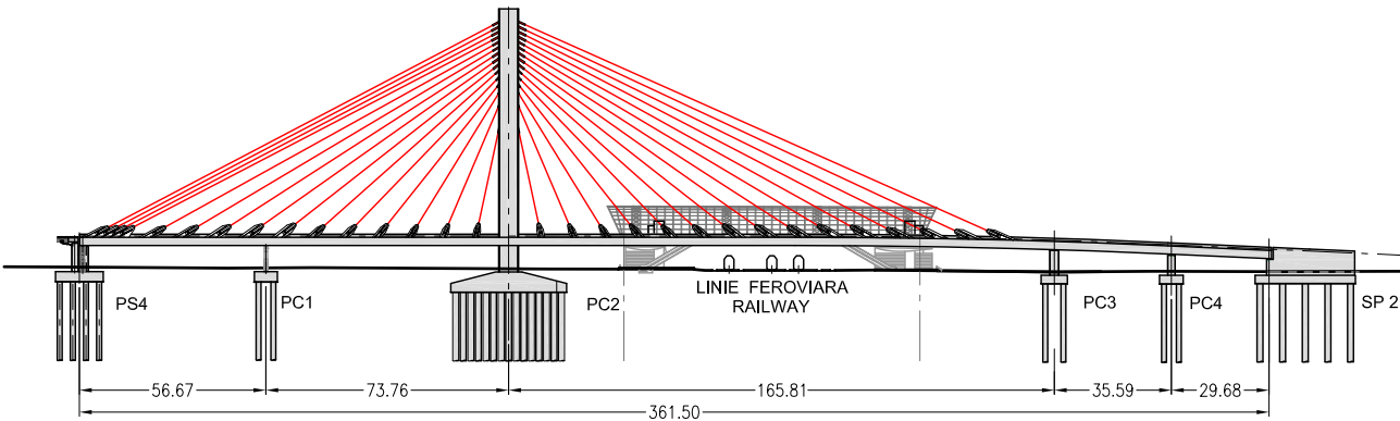
ALZADO GENERAL POR EJE ESCALA 1:2500
