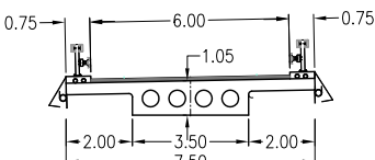
SECCION POR RAMPA ESCALA 1:500
