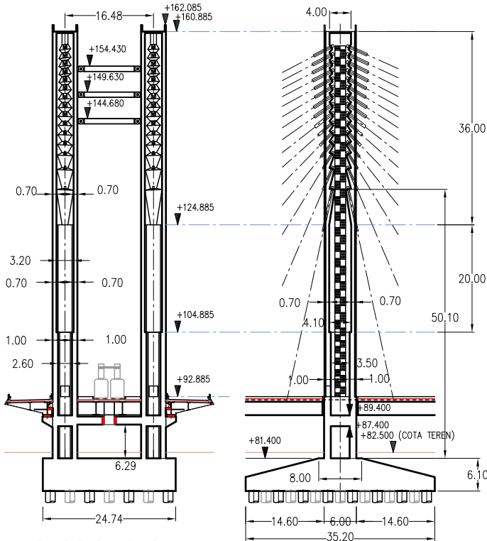
SECCION (VISTA FRONTAL) ESCALA 1:1000
