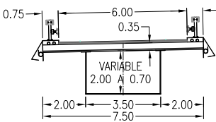
SECCION POR RAMPA ESCALA 1:500
