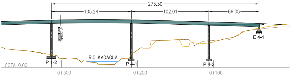
ALZADO DE VIADUCTO 4 ESCALA 1:3000
