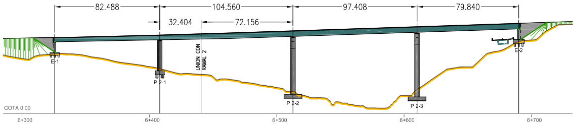
ALZADO DE VIADUCTO 2 ESCALA 1:3000
