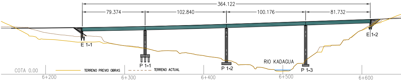
ALZADO DE VIADUCTO 1 ESCALA 1:3000
