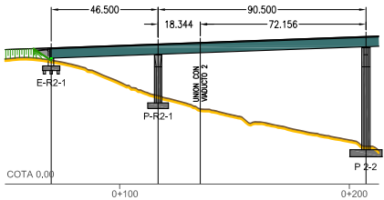
ALZADO DE RAMAL 2 ESCALA 1:2000
