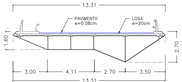
SECCIÓN 2-2 ESCALA 1:200
