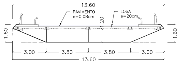
SECCIÓN 3-3 ESCALA 1:200
