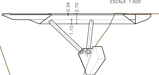
SECCIÓN 1-1 ESCALA 1:500
