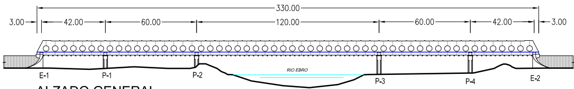
ALZADO GENERAL ESCALA 1:2500
