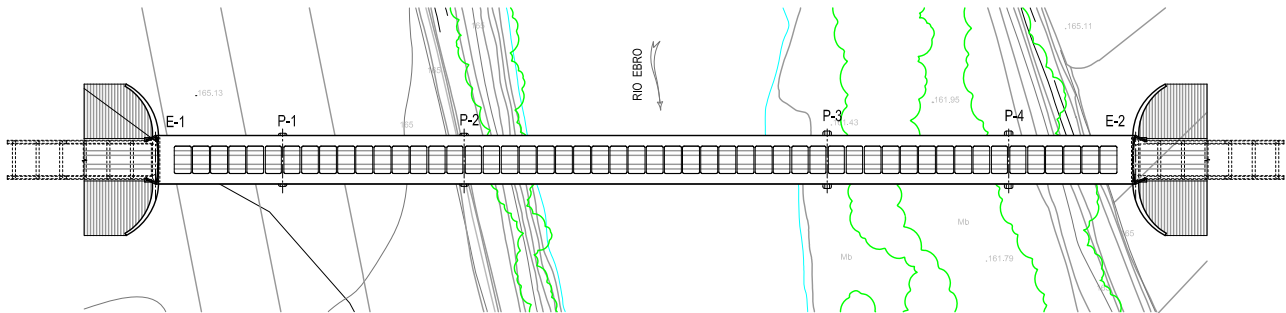
PLANTA GENERAL ESCALA 1:2500
