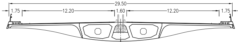
SECCION TRANSVERSAL POR ANCLAJES DE TIRANTES
