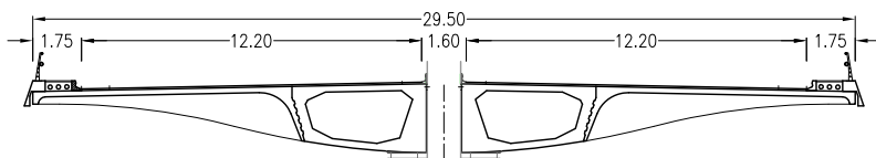
SECCION TRANSVERSAL POR TORRE
