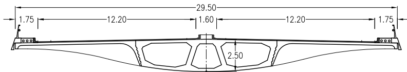
SECCION TRANSVERSAL TIPO
