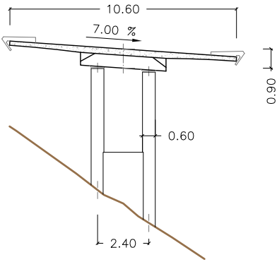
ALZADO FRONTAL PILA 1 ESCALA 1:250
