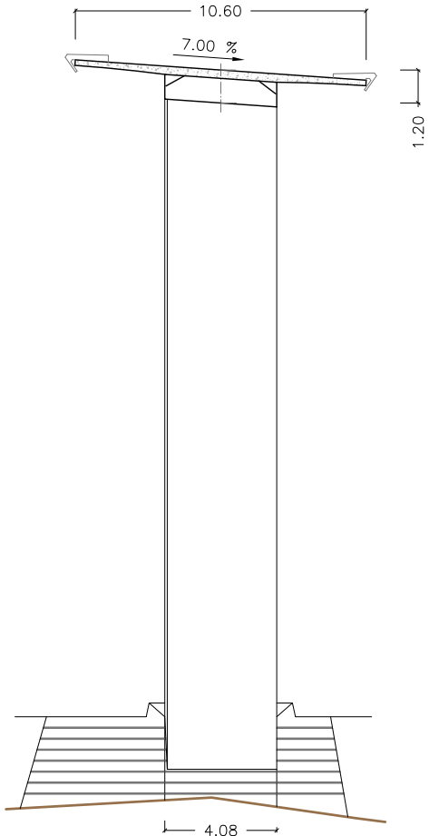
ALZADO FRONTAL PILA 2 ESCALA 1:250
