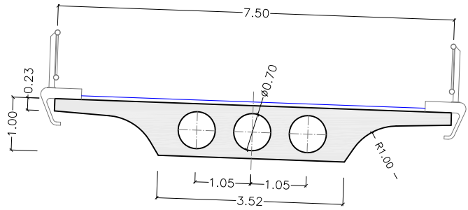
SECCIÓN TRANSVERSAL POR CENTRO DE VANO ESCALA 1:100
