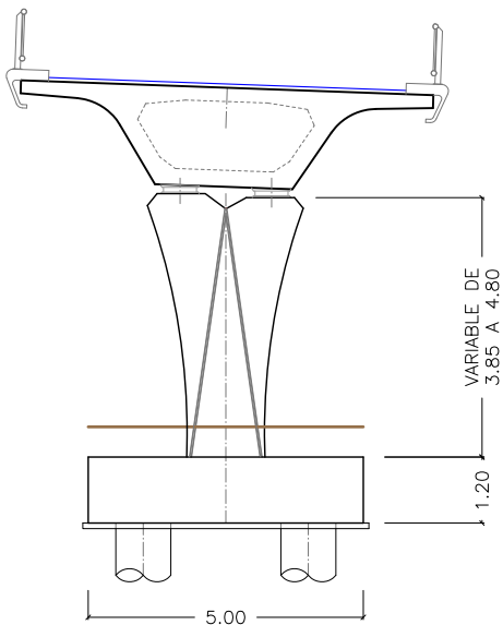
ALZADO DE PILAS ESCALA 1:150
