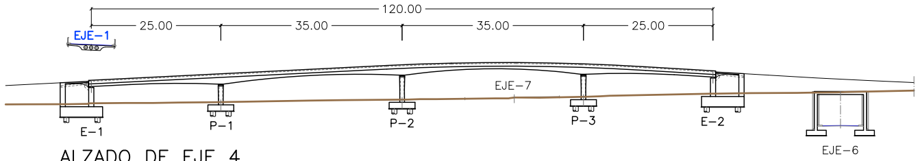
ALZADO DE EJE 4 ESCALA 1:1000
