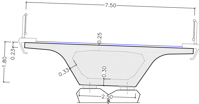
SECCIÓN TRANSVERSAL POR PILA ESCALA 1:100
