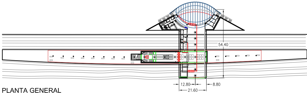
PLANTA GENERAL ESCALA 1:1500
