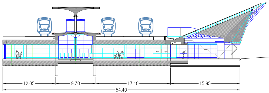
SECCION TRANSVERSAL ESCALA 1:500
