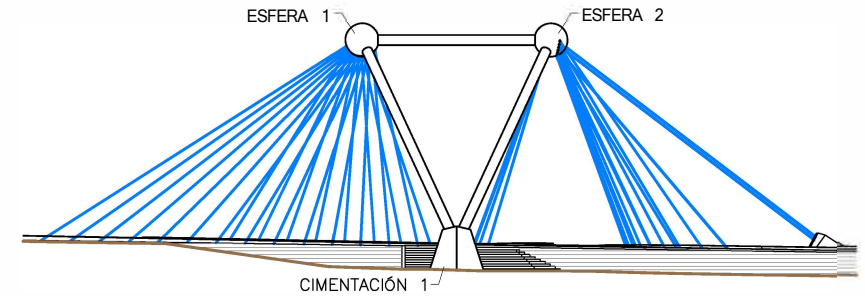
VISTA POR A ESCALA 1:500
