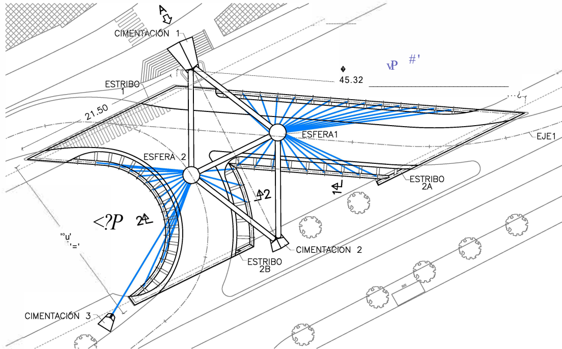
PLANTA SUPERIOR GENERAL ESCALA 1:500
