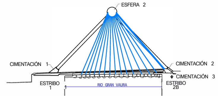
VISTA POR B ESCALA 1:500
