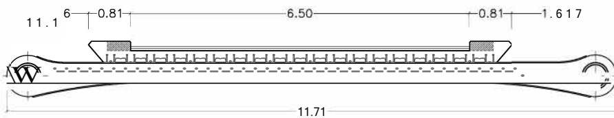
SECCIÓN 2-2 ESCALA 1:100
