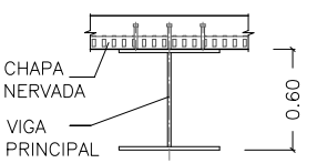
SECCIÓN 2-2 ESCALA 1:50
