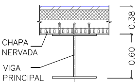
SECCIÓN 1-1 ESCALA 1:50
