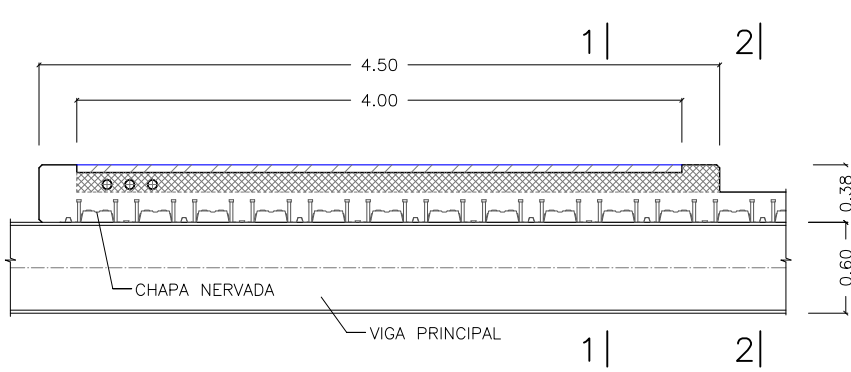
SECCIÓN TIPO ESCALA 1:50
