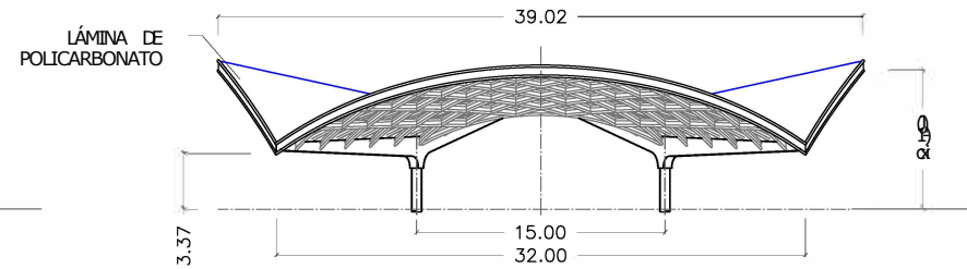
ALZADO FRONTAL VISTO POR B ESCALA 1:500
