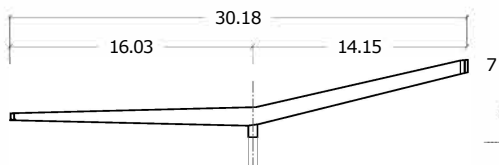
ALZADO DE VIGA PRINCIPAL ESCALA 1:500
