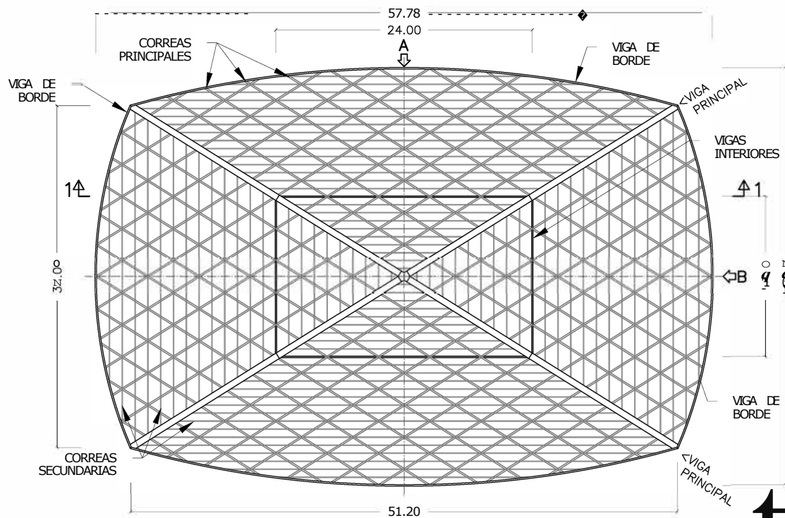
ESTRUCTURA DE CUBIERTA. PLANTA SUPERIOR ESCALA 1:500
