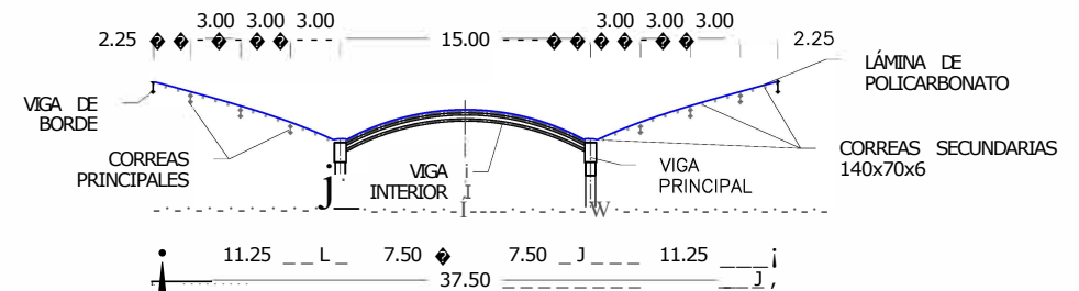
SECCIÓN 1-1 ESCALA 1:500
