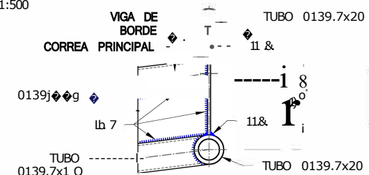
SECCIÓN DE VIGA DE BORDE ESCALA 1:25
