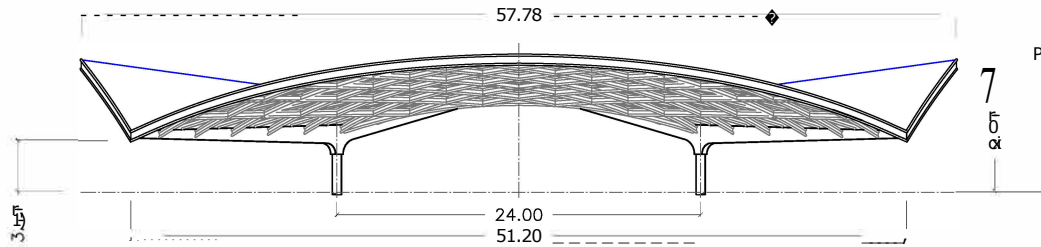
ALZADO FRONTAL VISTO POR A ESCALA 1:500
