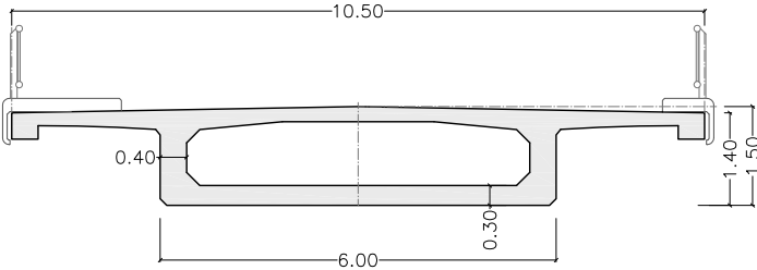
SECCIÓN TRANSVERSAL POR TABLERO ESCALA 1:125
