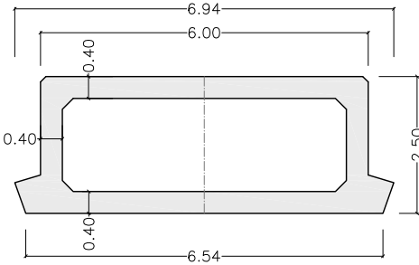
SECCIÓN TRANSVERSAL POR ARCO ESCALA 1:125
