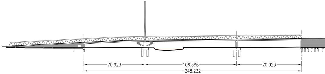
ALZADO GENERAL ESCALA 1:2500
