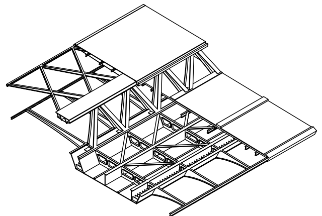
AXONOMETRICA TABLERO ESCALA 1:500
