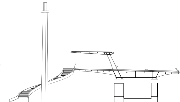
SECCION TRANSVERSAL POR PILA 1 Y ESCALERA ESCALA 1:500
