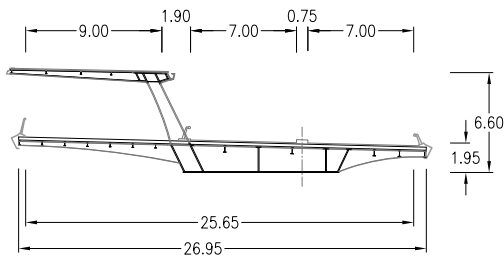
SECCION TRANSVERSAL TIPO ESCALA 1:500
