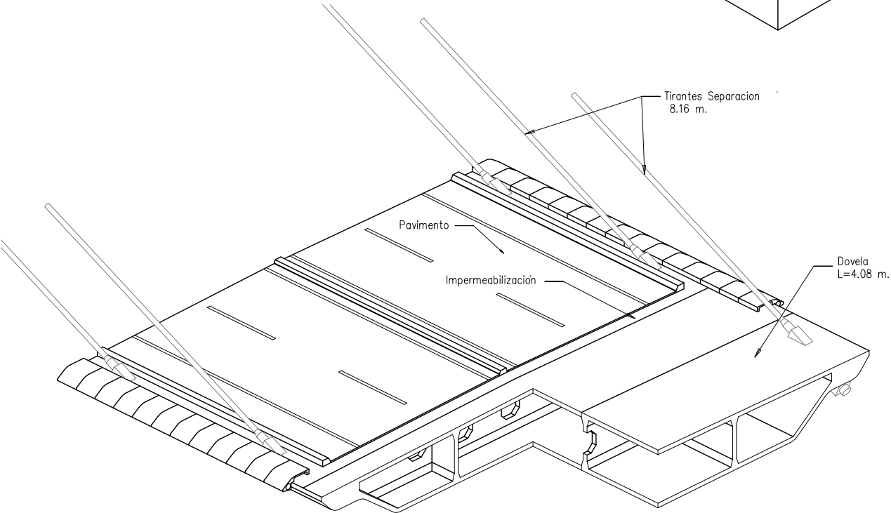
PERSPECTIVA SECCION TABLERO
