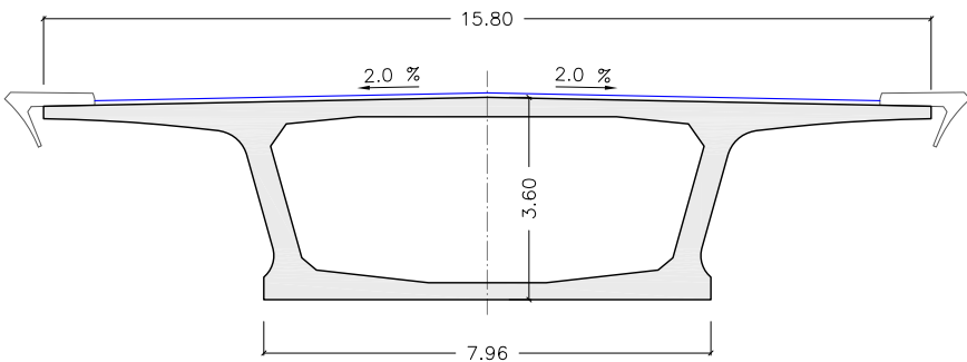
SECCIÓN TRANSVERSAL POR CENTRO DE VANO ESCALA 1:150
