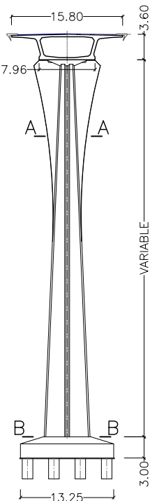
ALZADO FRONTAL DE PILAS ESCALA 1:750
