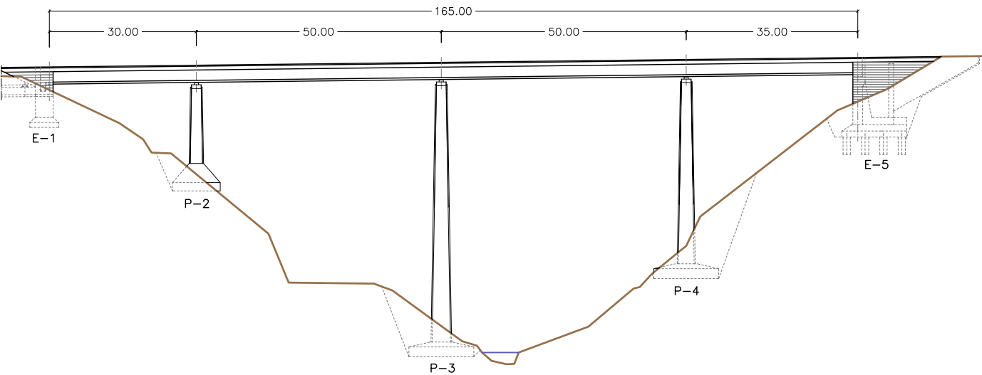
ALZADO LONGITUDINAL ESCALA 1:1100
