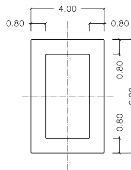
SECCIÓN B-B ESCALA 1:200
