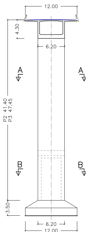
SECCIÓN TRANSVERSAL POR PILA ESCALA 1:500
