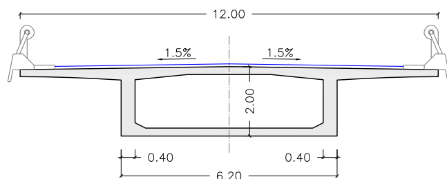
SECCIÓN TRANSVERSAL TIPO ESCALA 1:150
