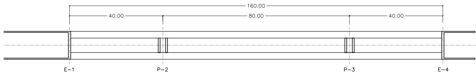
PLANTA INFERIOR ESCALA 1:1000
