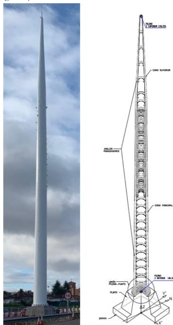
Figura 6. Pilono.
