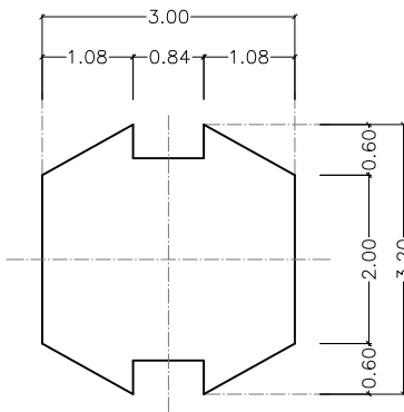
SECCIÓN TRANSVERSAL TIPO ESCALA 1:100
