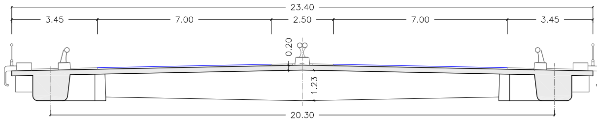
SECCIÓN TRANSVERSAL TIPO ESCALA 1:150
