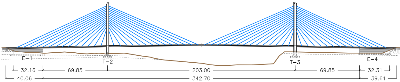
ALZADO GENERAL ESCALA 1:2500
