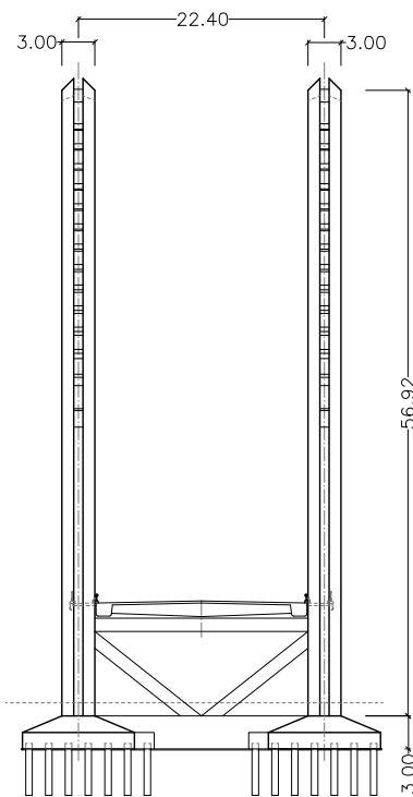
ALZADO FRONTAL DE LA TORRE ESCALA 1:750
