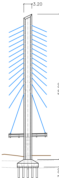
ALZADO LATERAL ESCALA 1:750
